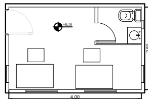
Esquema de Estación de Pesaje Esc.: 1:75
